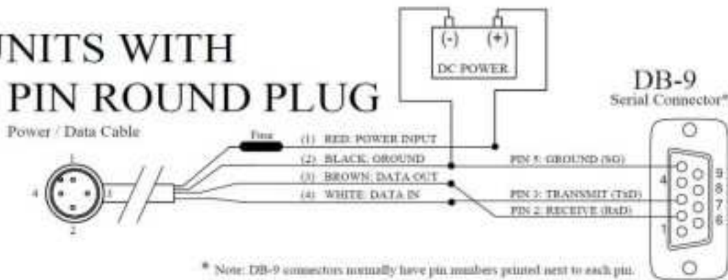
Connexion du GPS 72H à un appareil standard NMEA 0183
