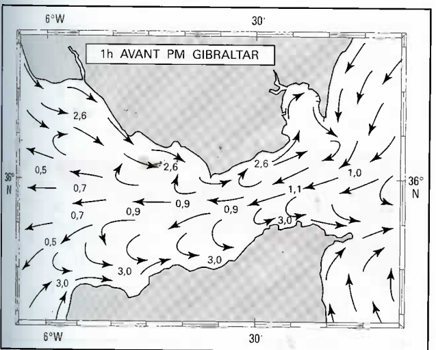
1.0.2.3.A. — Courants de marée dans le Déroit de Gibraltar.
