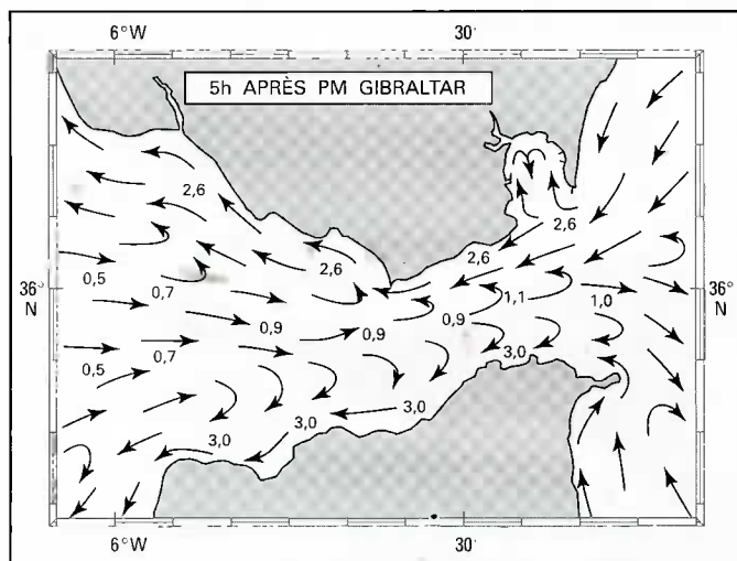
1.0.2.3.B. — Courants de marée dans le Déroit de Gibraltar.
