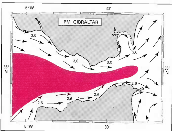
1.0.2.3.A. — Courants de marée dans le Déroit de Gibraltar.
