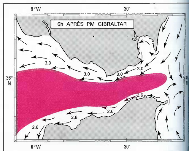
1.0.2.3.B. — Courants de marée dans le Déroit de Gibraltar.
